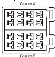
Расположение контактов разъема ISO:
